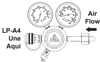
Módulo de Prueba de Calidad del Aire del Compresor de Baja Presión
